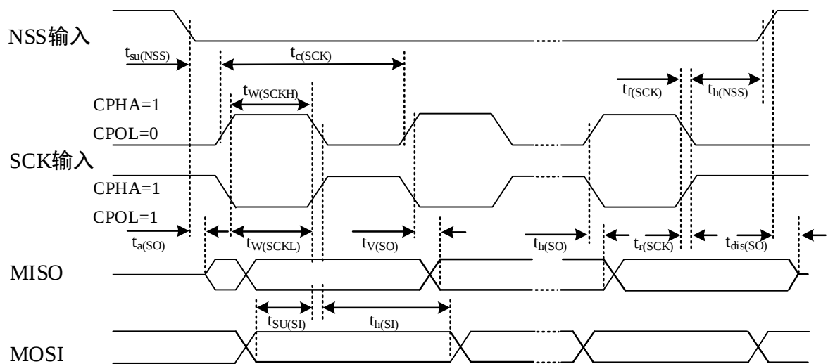
图 4-3 SPI 从模式时序图 (CPHA=1) (1)
